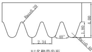
PJ多楔带齿形
