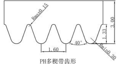
PH多楔带齿形
