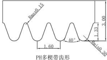
PH多楔带齿形
